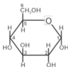
\alpha -D(+)-Glucose
