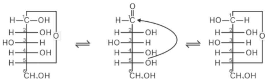
\alpha -D(+)-Glucose
