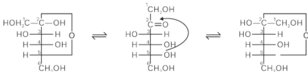
\alpha -D(-)-Fructofuranose
