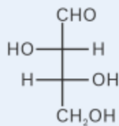
D-Threose
