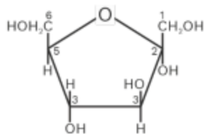
\alpha -D(-)-Fructofuranose
