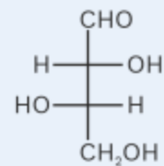
L-Threose
