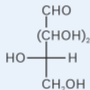
L-Aldopentose
