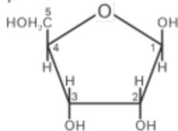
\beta -D-ribose
