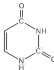
Uracil (U)
