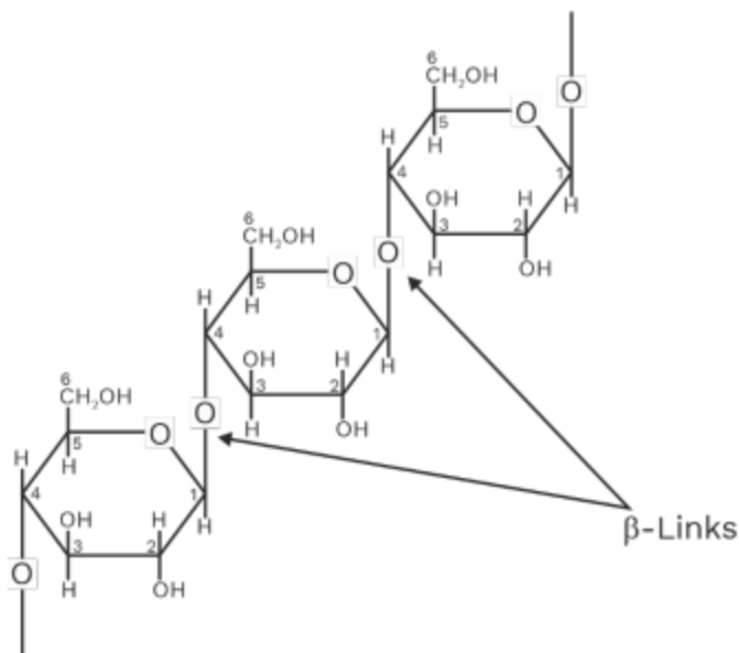
Cellulose
