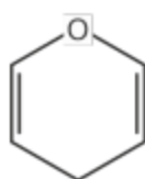
Pyran
