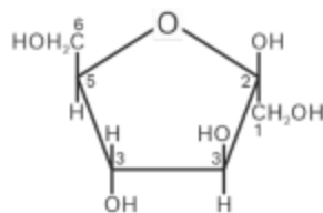
\beta -D(-)-Fructofuranose
